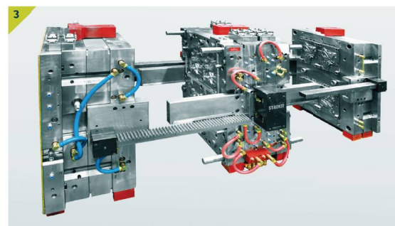
1 3-component precision mold 三物料模具
