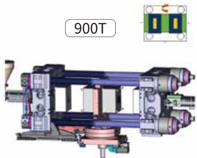
对射水平转盘注塑成型
